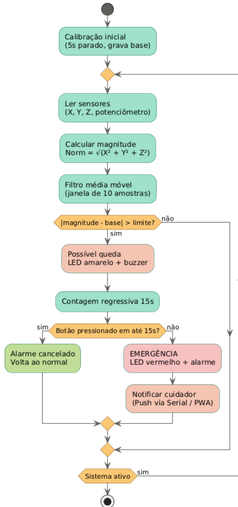
Figura 2 – Fluxograma do funcionamento do sistema SMN-Q.
