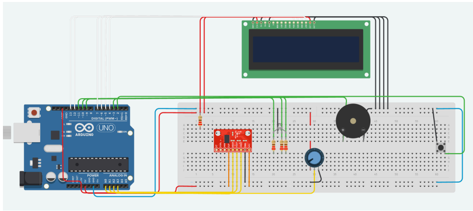
Figura 1 – Circuito do SMN-Q montado na plataforma Tinkercad.
